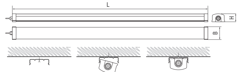
Рис.2 Схема монтажа светильника
